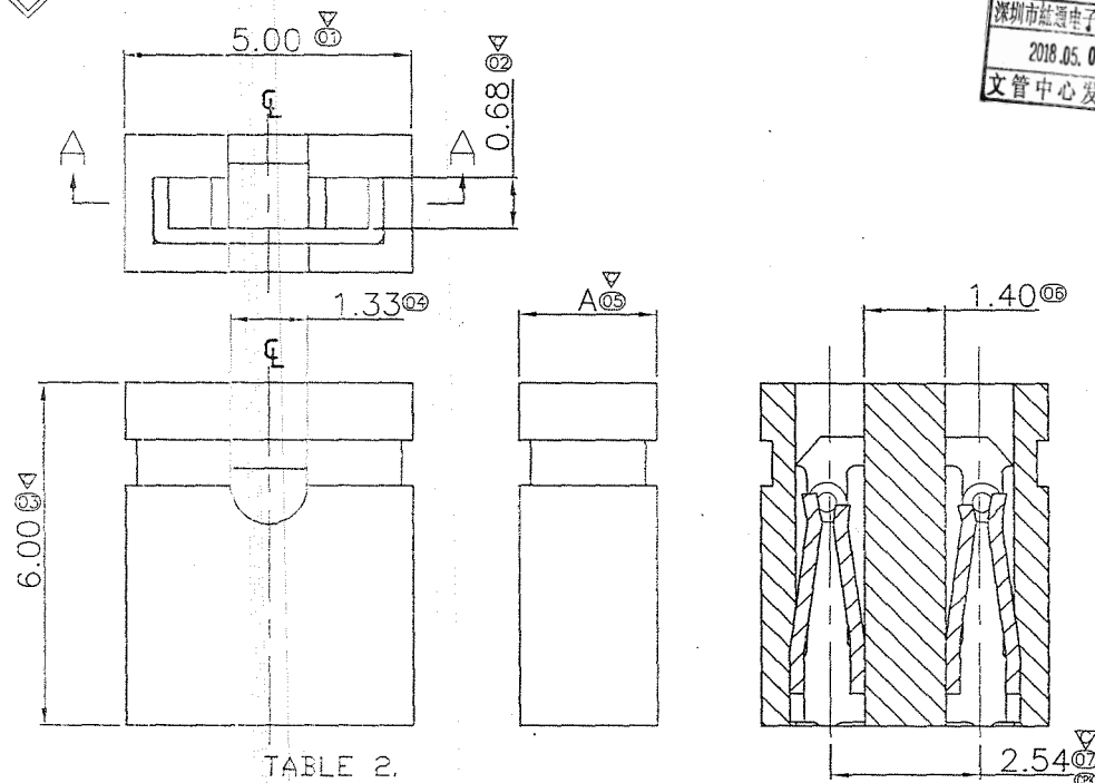
SEC:A-A
