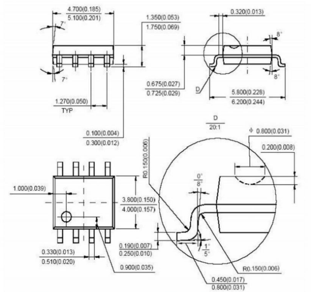
封装尺寸图 (SOP8)
