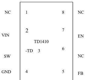
图(1) XL1410-TD封装
