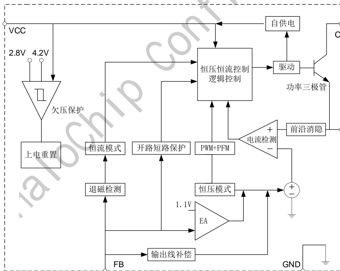
图 3 GP8891X 内部框图
