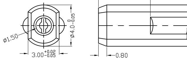
轴心部尺寸详图
