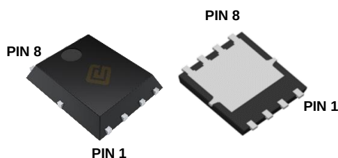
PDFN5*6
