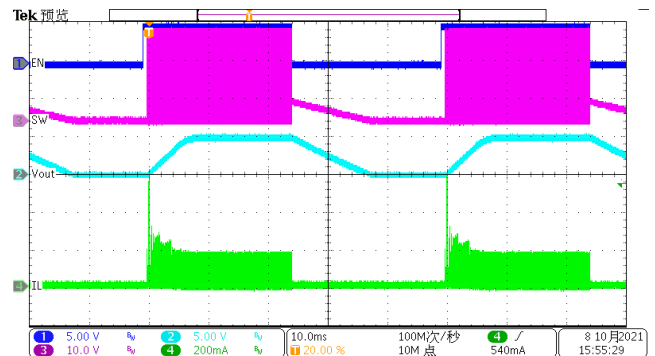
Figure 14. EN toggle (Iload=10mA)
