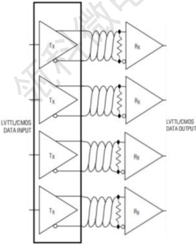
图 1 典型应用框图
