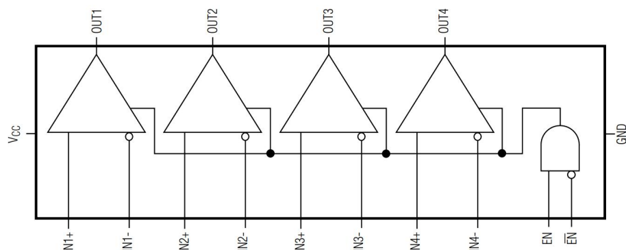
图 3 功能框图
