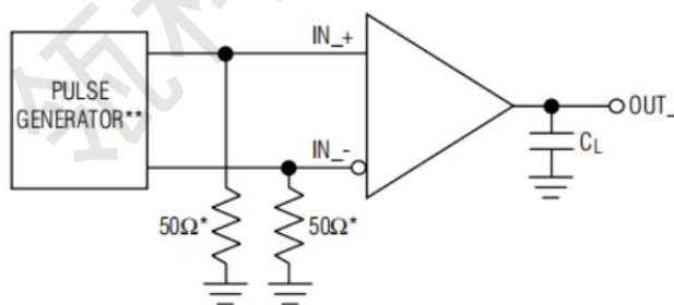
图 5 接收器传输延时测试电路
