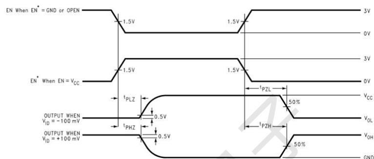
图 8 时序图 (三态传输延时)
