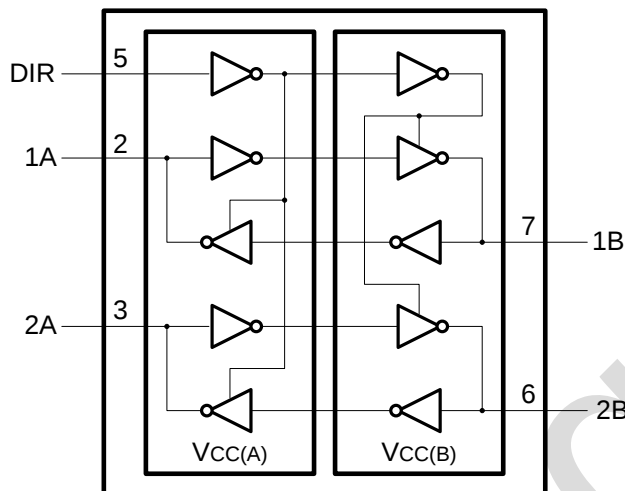
图 1 逻辑符号
