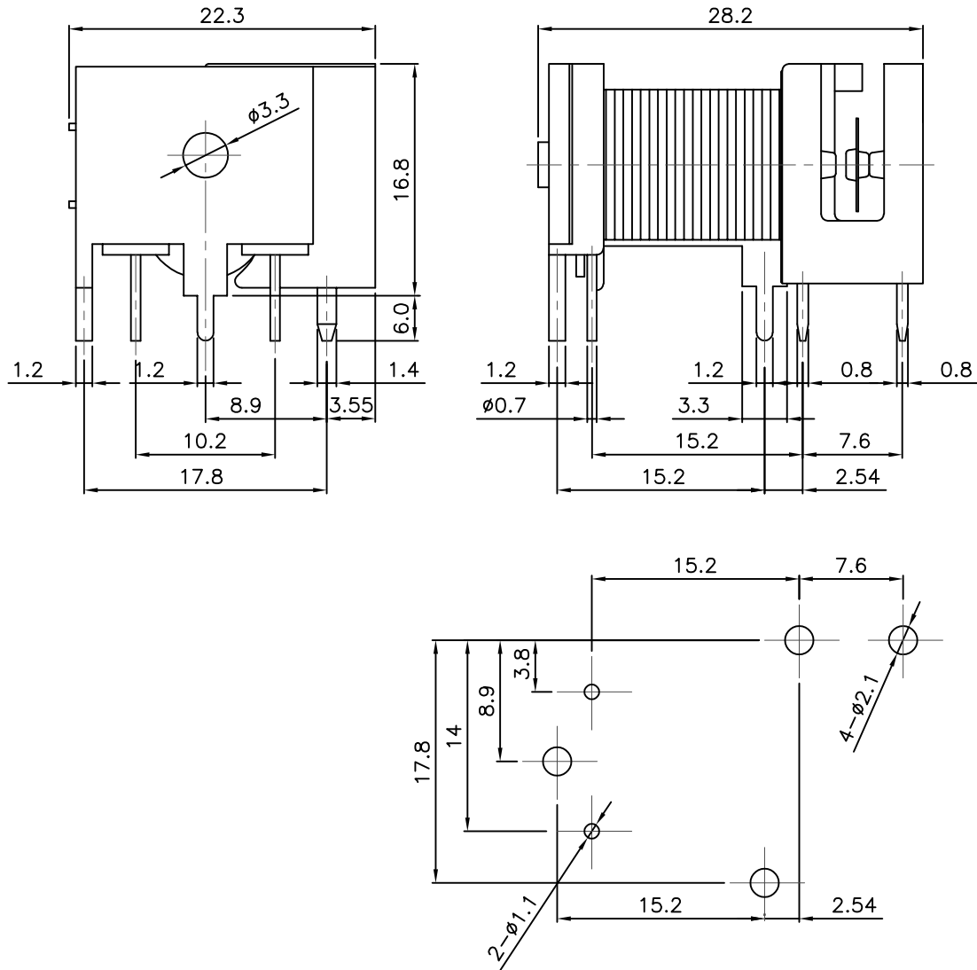
P.C.B LAYOUT
