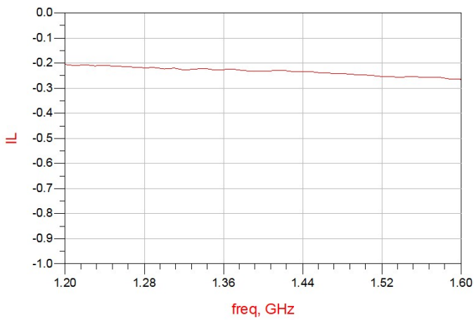
Figure 10. MHC1400L03 IL
