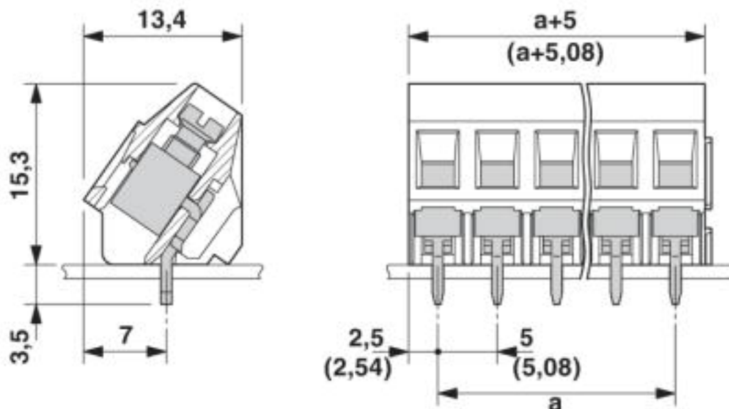
尺寸图
