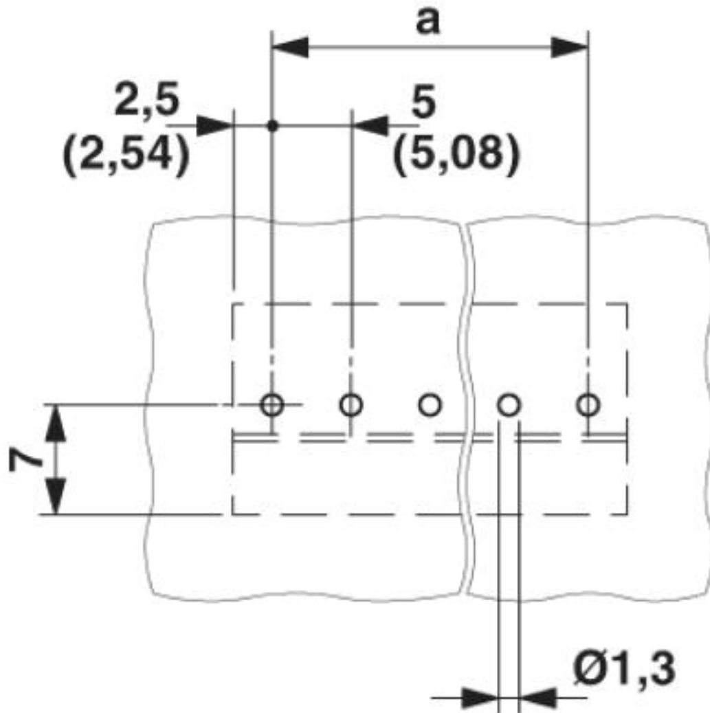
钻孔图
