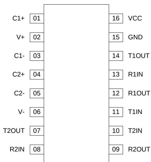
SOP -16 PKG
