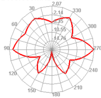
2400.000MHz E1
