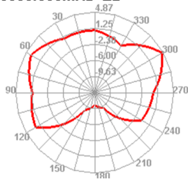
5850.000MHz E2
