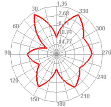
5150.000MHz E1
