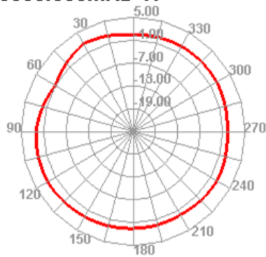
5850.000MHz H
