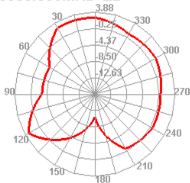
5500.000MHz E2
