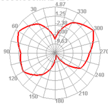
5850.000MHz E1
