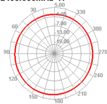
2400.000MHz H
