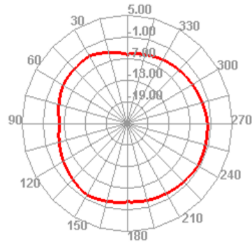
5150.000MHz H
