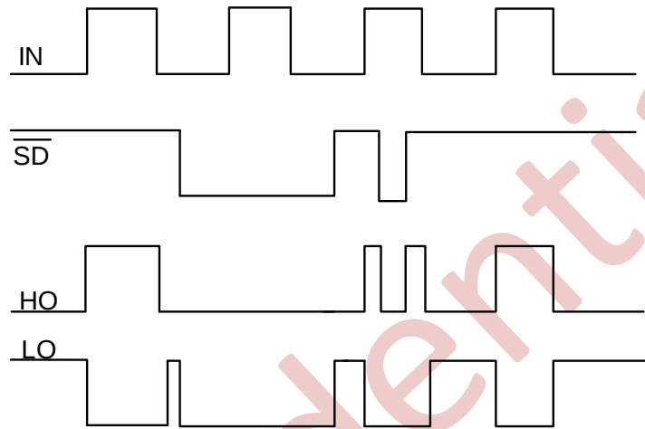
图 9-1 NSG6002 输入输出时序波形
