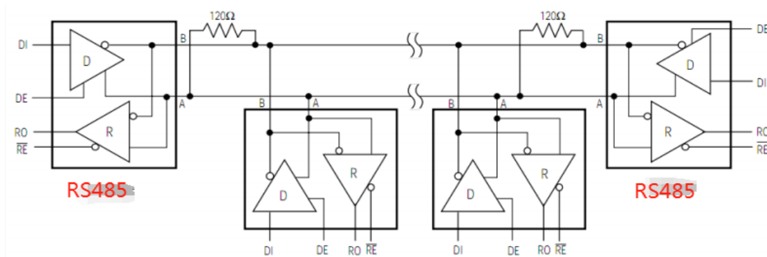
图 11 典型的 RS485 半双工通讯网络
