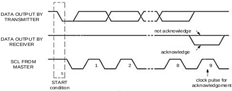
图 5-10 I2C 总线的数据传输
