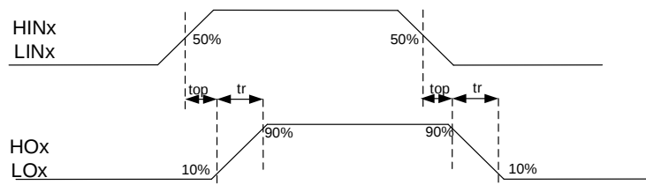
图 5-4 开关时间
