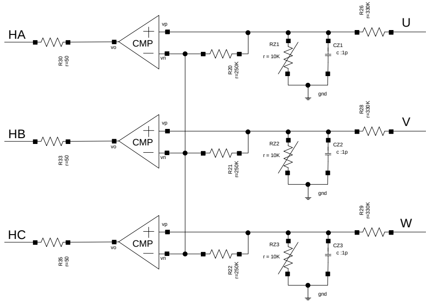
图 5-13 过零检测内部电路框图
