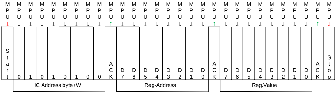
图 5-11 写命令格式
