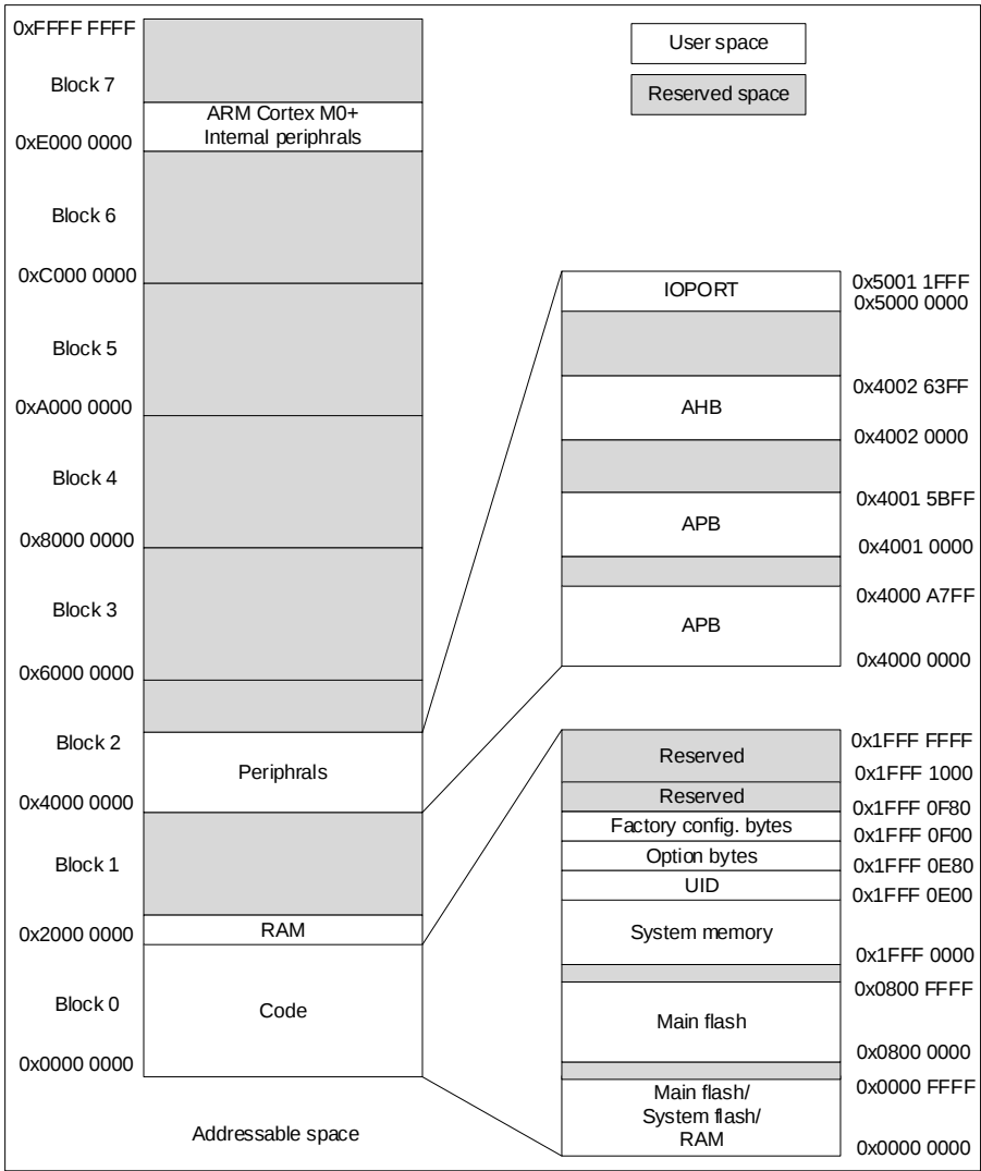
图 4-1 存储器映射
