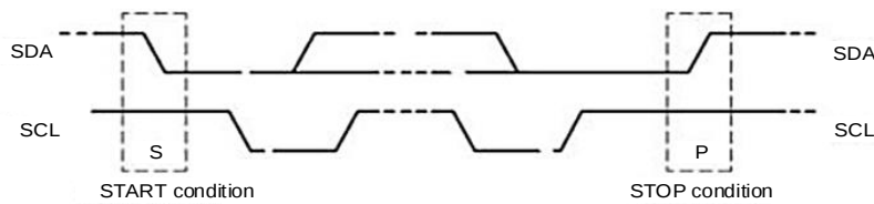
图 5-7 起始和停止条件
