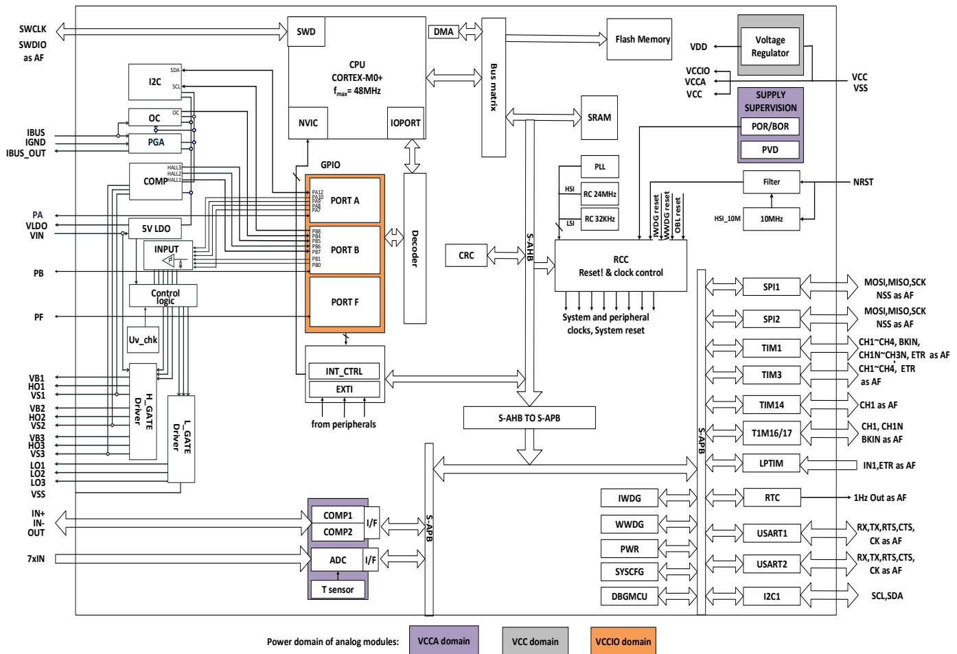
图 1-1 功能模块
