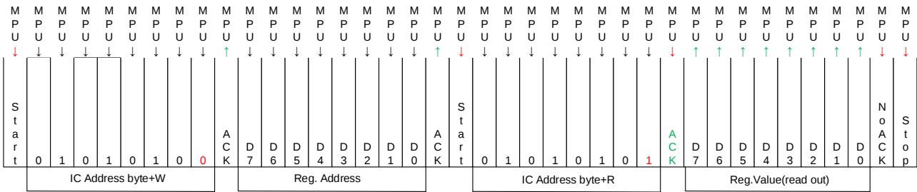
图 5-12 读命令格式
