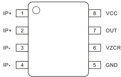
SOP8 Package
