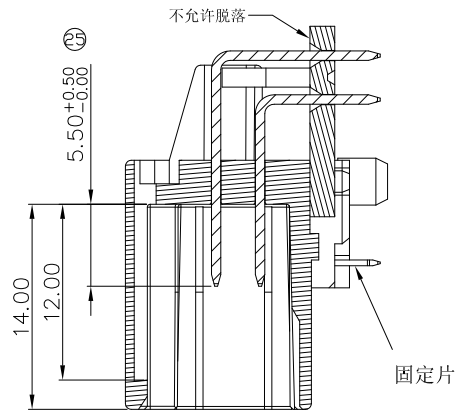
剖视图 A-A
