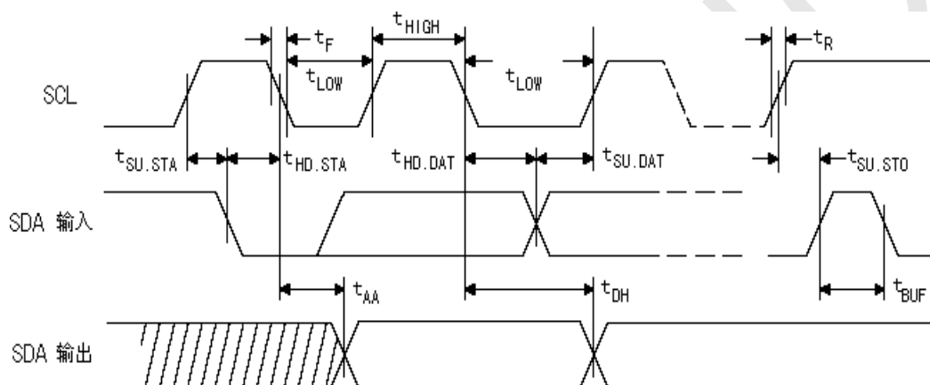
图 5、总线时序
