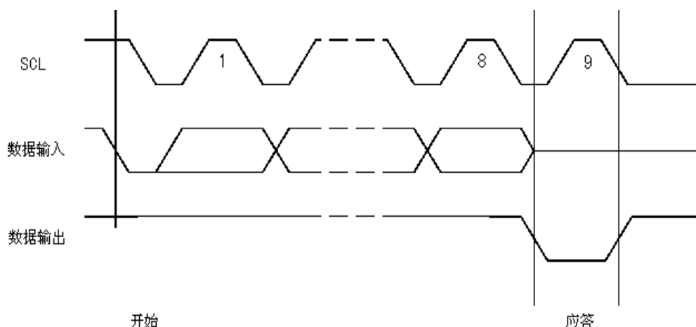
图 7、输出响应
