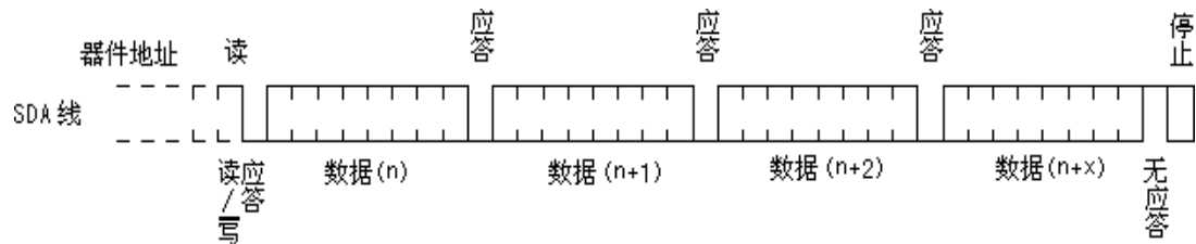
图 12、顺序地址读操作
