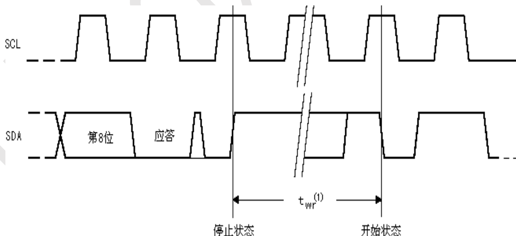
图 6、写周期时序
