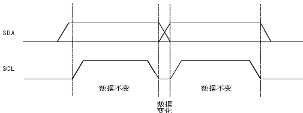
图 3、数据有效时序图
