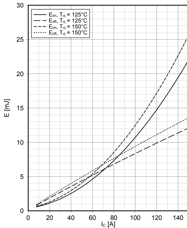
スイッチング損失 IGBT- インバータ (Typical) switching losses IGBT, Inverter (typical)
