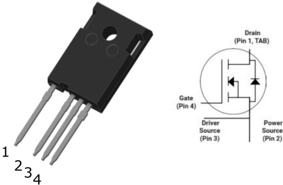
TO-247-4L
