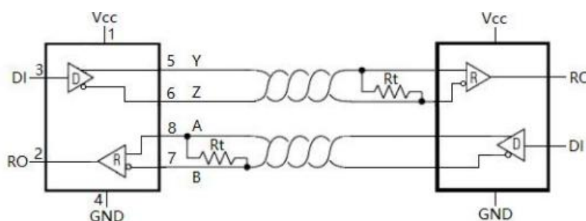
图 3: HX490E 典型全双工应用电路
