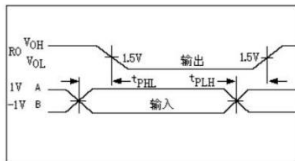
图 7: 接收器传播延时
