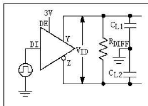
图 5: 驱动器时序测试电路
