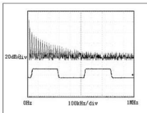
图 9: 传输 20kHz 信号时 HX490E 驱动器输出波形 FFT 图
