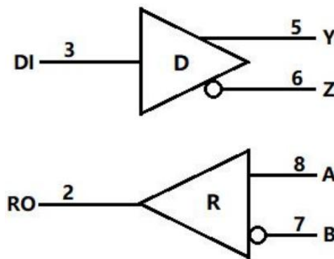
图 2: HX490E 逻辑图
