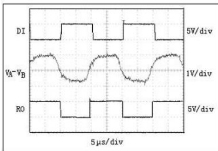
图 10: 在 50kHz 时驱动 4000 英尺的电缆 HX490E 系统差分电压线性转发器
