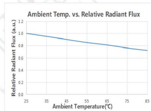
4) 环境温度与相对辐射通量特性曲线
