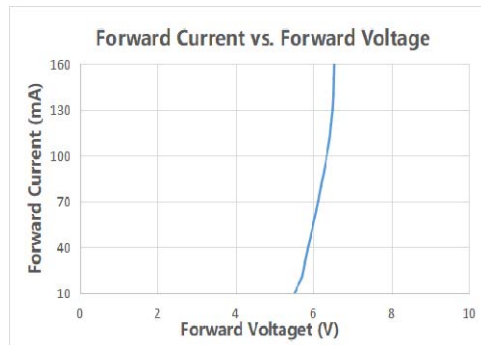
1) 伏安特性曲线
