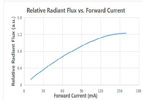
2) 正向电流与相对辐射通量特性曲线
