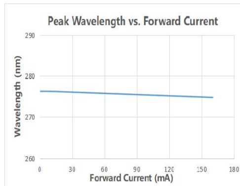
3) 正向电流与峰值波长特性曲线
