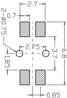
PCB线路板图
