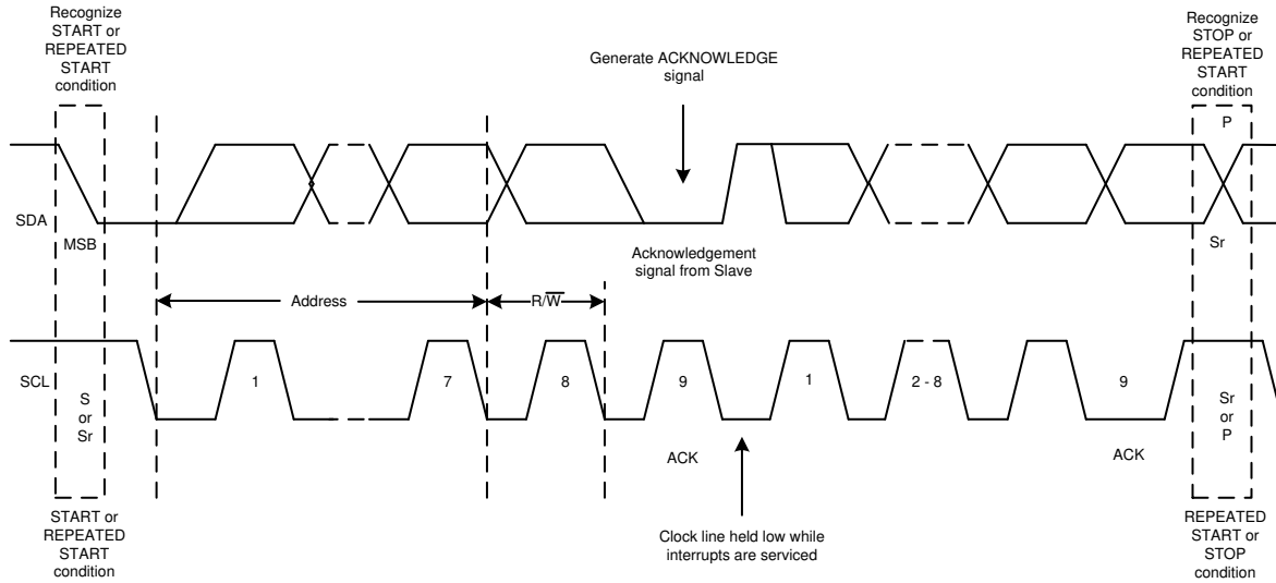
图 7-5. I 2 C Bus Protocol
