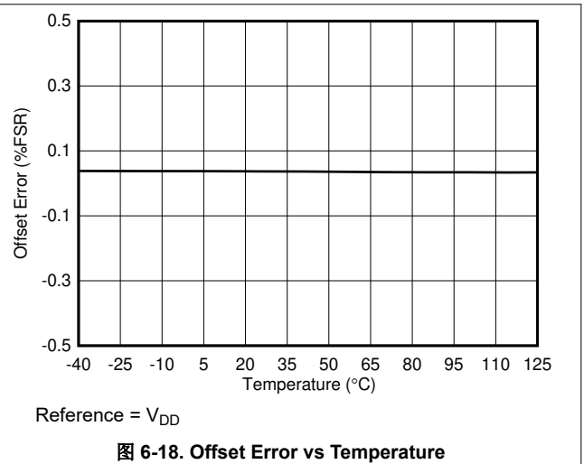
图 6-18. Offset Error vs Temperature
