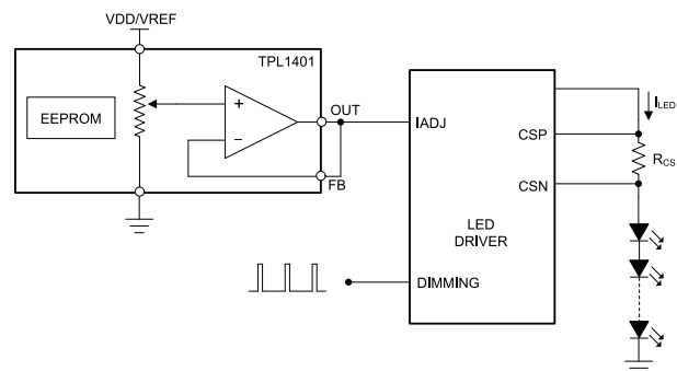
通过 TPL1401 实现可编程电流限制
