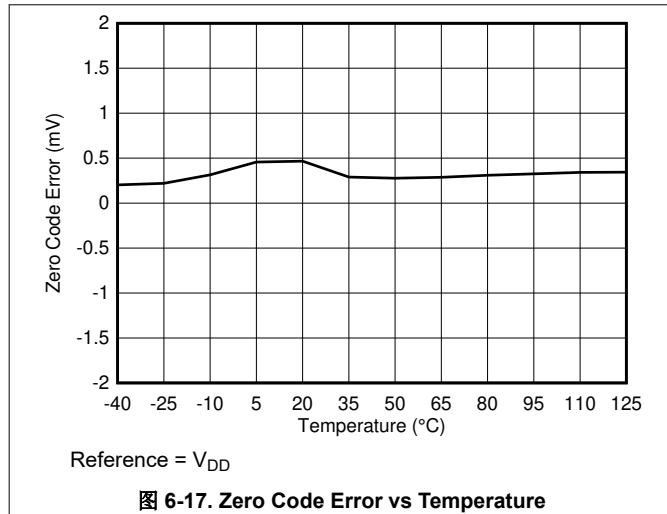
图 6-17. Zero Code Error vs Temperature
