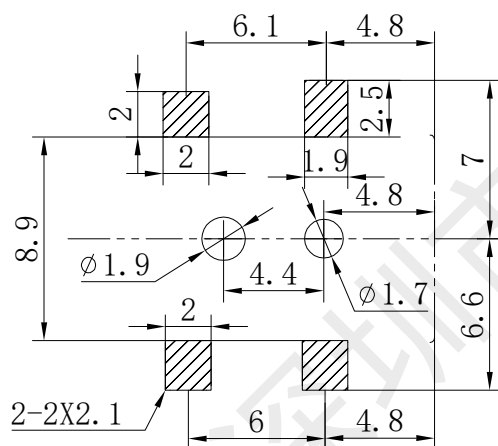
线路板开孔尺寸 P.C.B LAYOUT
