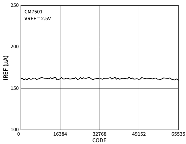
图 10 IREF 随 CODE 的变化 (CM7501)
