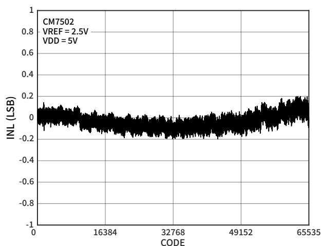
图 2 INL 误差 (CM7502)
