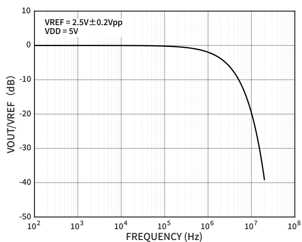
图 19 VOUT/VREF
