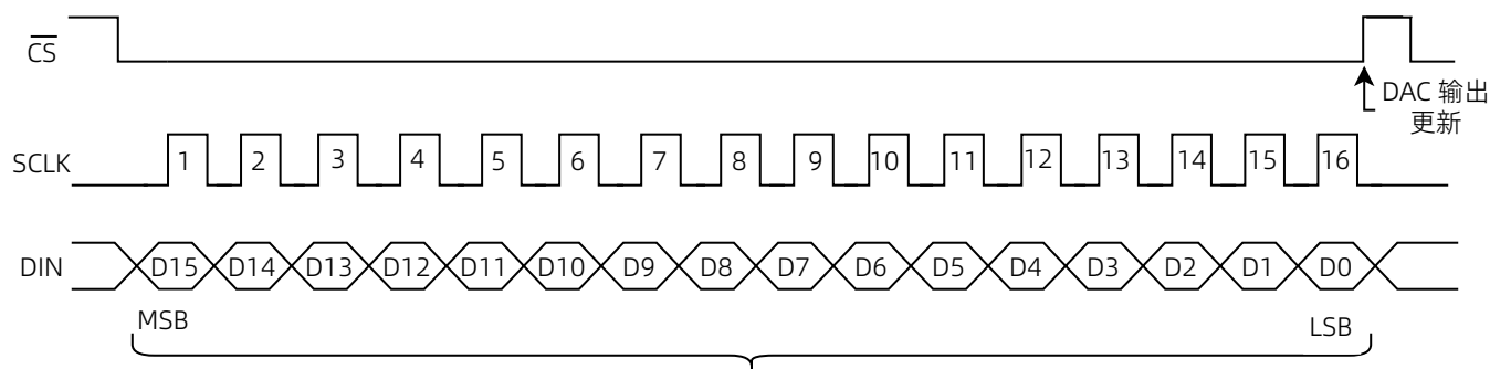
图 28 时序图
