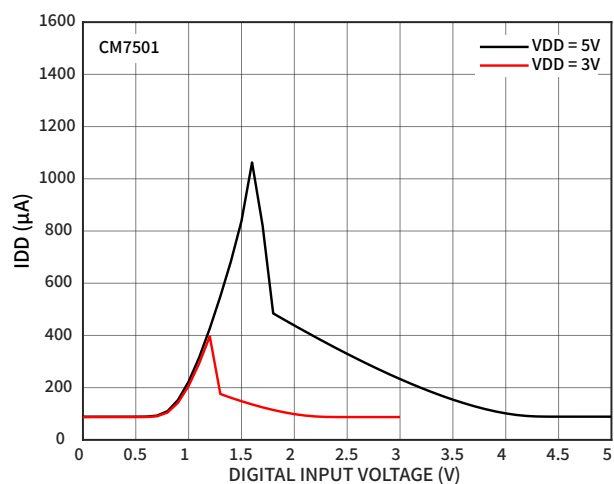
图 14 IDD 随 VIH 的变化 (CM7501)
