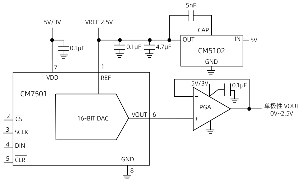
图 30 典型连接 (CM7501)
