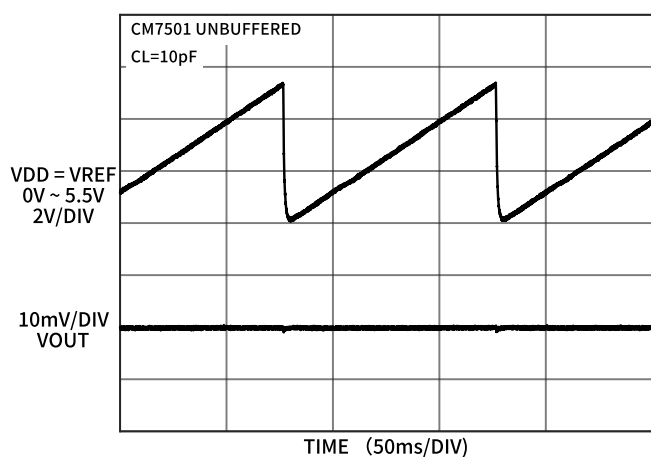
图 18 VOUT 随上电时间的变化 (上电复位功能, CM7501)
