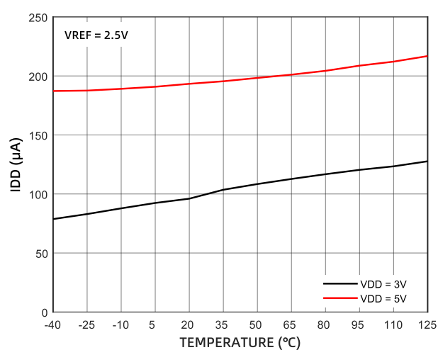
图 17 IDD 的温度特性 (上电复位功能, CM7501)
