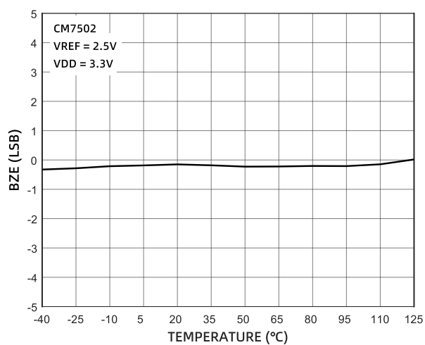
图 26 0 码误差的温度特性 (CM7502)
