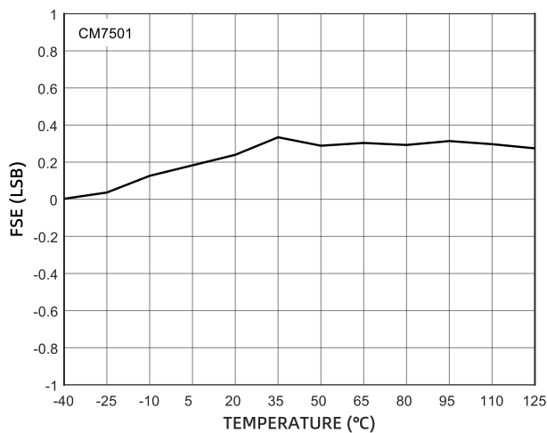
图 24 满量程误差的温度特性 (CM7501)
