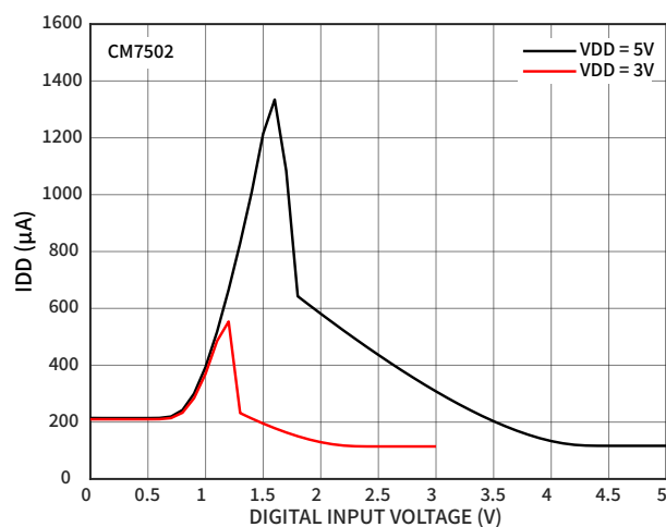
图 15 IDD 随 VIH 的变化 (CM7502)
