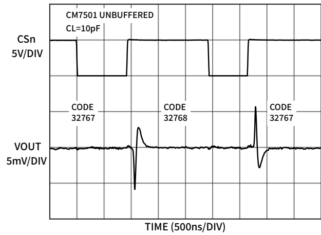
图 21 主进位翻转毛刺脉冲 (CM7501)
