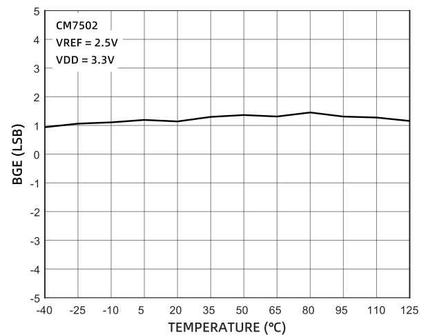
图 25 增益误差的温度特性 (CM7502)
