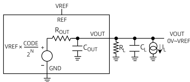
图 27 VOUT 管脚等效电路
