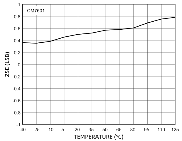
图 23 0 码失调误差的温度特性 (CM7501)
