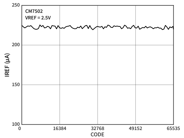
图 11 IREF 随 CODE 的变化 (CM7502)
