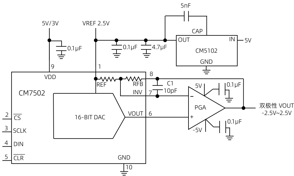
图 29 典型连接 (CM7502)
