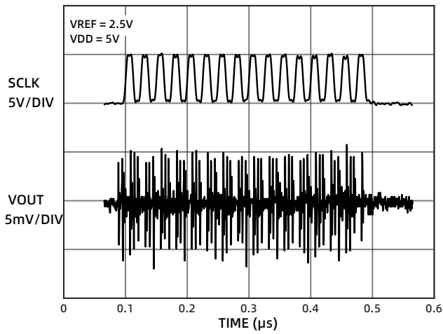
图 20 数字馈通
