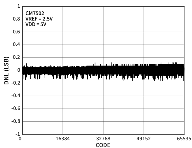
图 6 DNL 误差 (CM7502)
