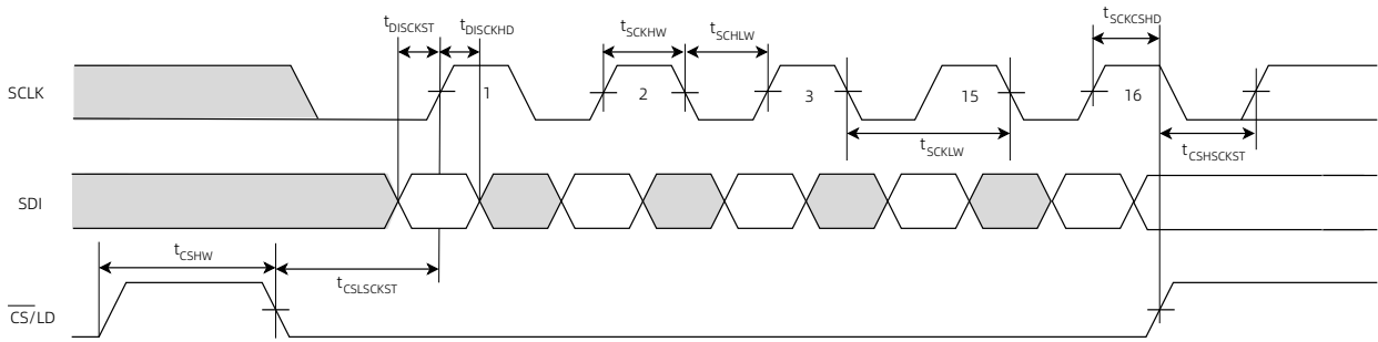
图 1 SPI 时序图
