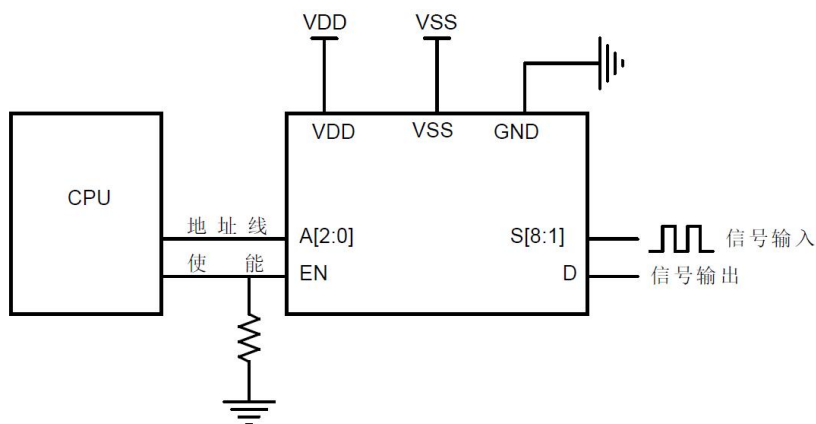
图 11 典型应用
