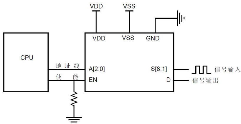
图 1 典型应用图
