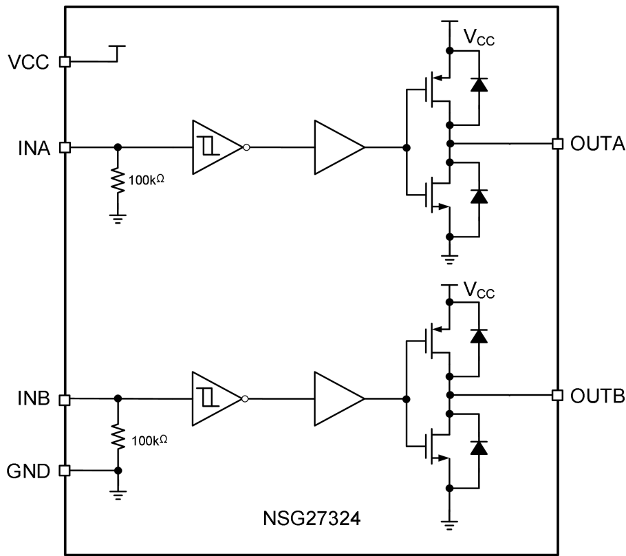
图 10-1 NSG27324P 功能框图
