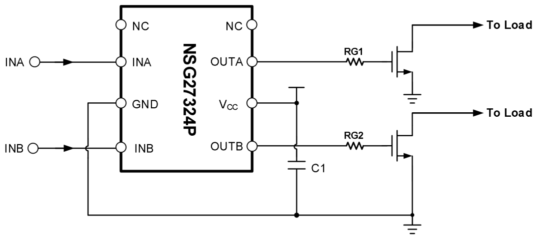
图 10-2 NSG27324P 典型应用电路图
