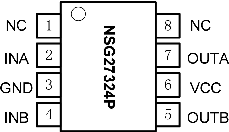
图 7-1 8-脚 DIP8 顶视图
