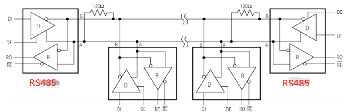
图 11 典型的 RS485 半双工通讯网络
