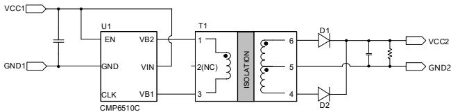
图3. CMP6510C 单路输出
