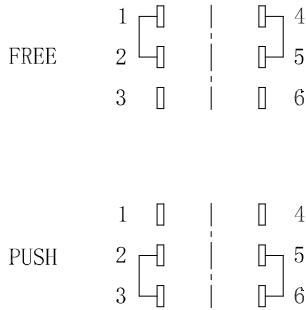
电路简示图
