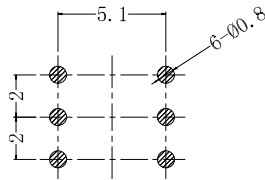
PCB参考图
