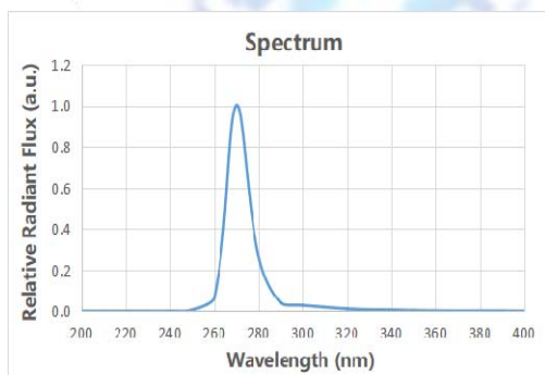
5) 光谱分布特性曲线
