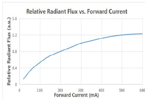
2) 正向电流与相对辐射通量特性曲线
