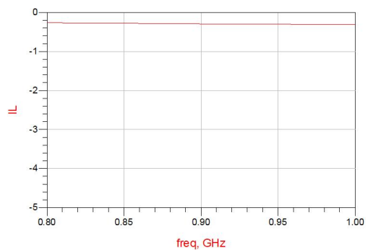
Figure 10. MHC0900M10 IL
