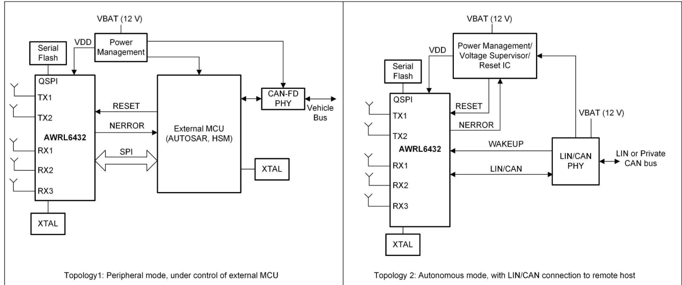
图 7-1. 系统拓扑
