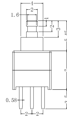
PCB参考图
