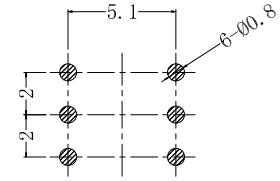
PCB参考图
