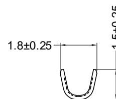
SECTION F1-F1
