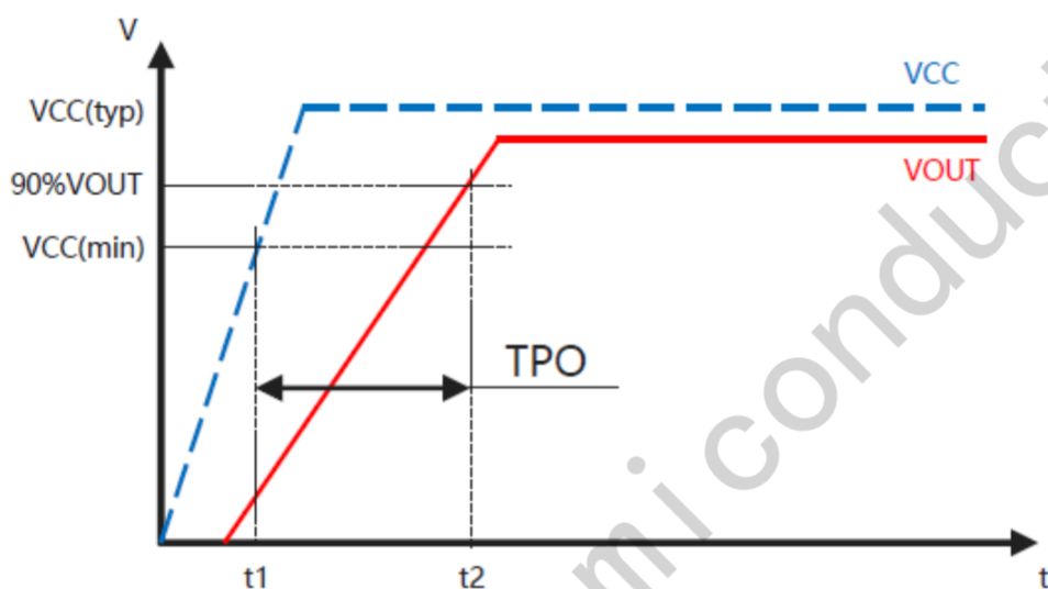
图 1：上电时间定义
