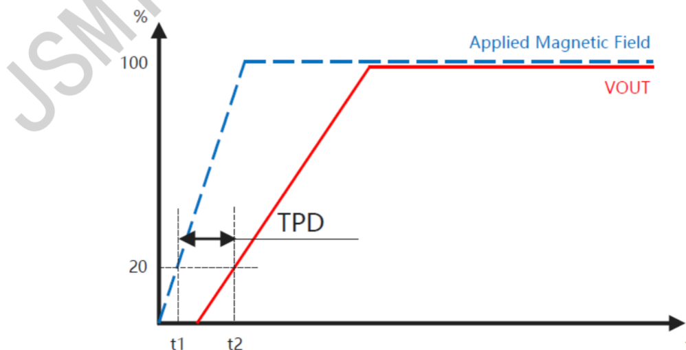
图 2：传输延迟定义
