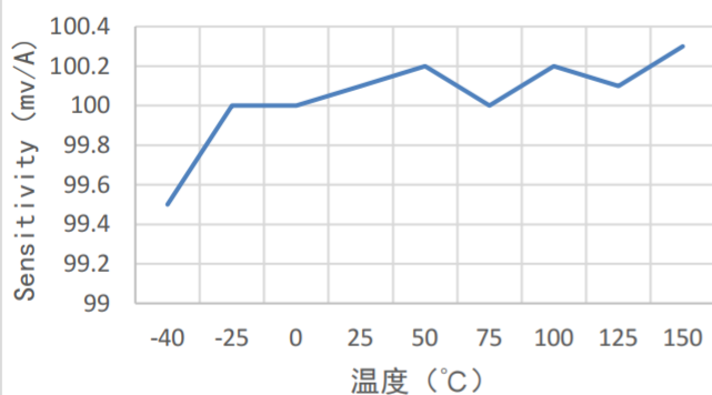
20A 灵敏度随温度变化
