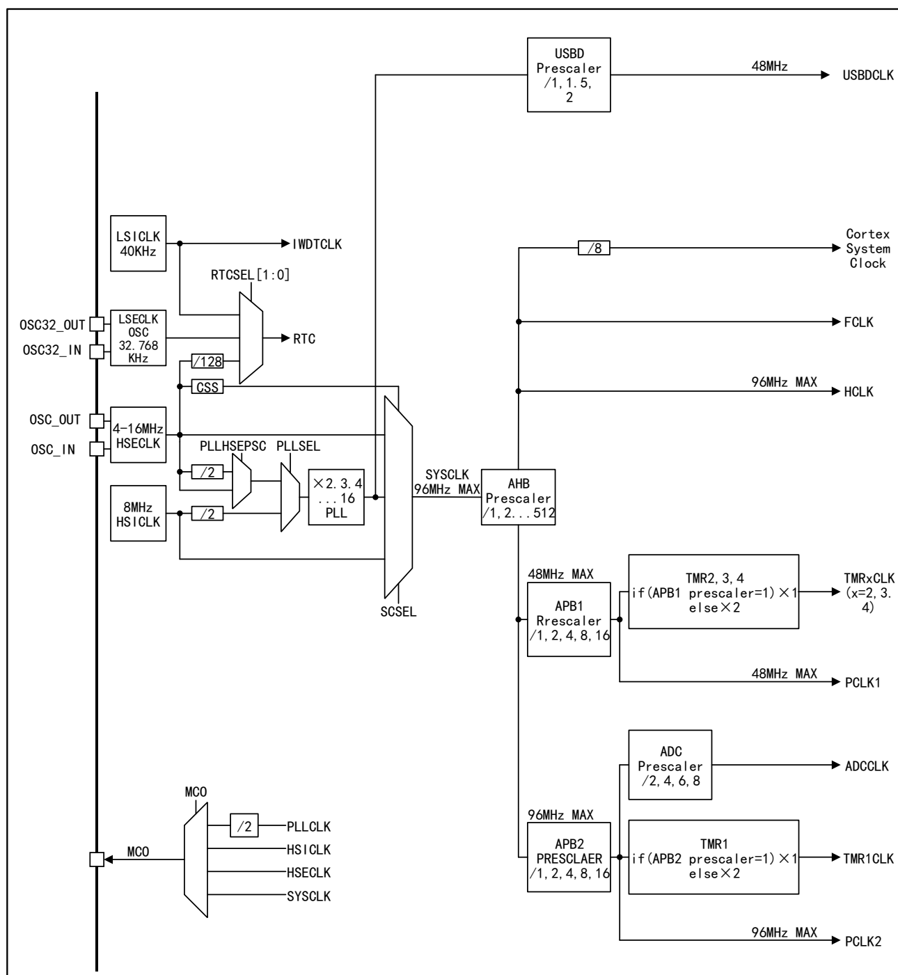
图 6 APM32F103x4x6x8 时钟树
