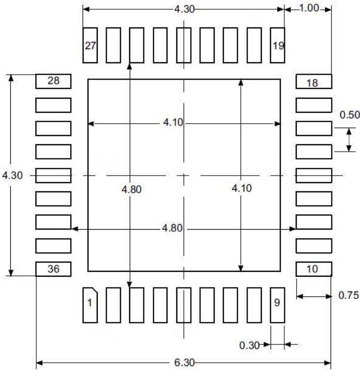
图 23 QFN36 焊接 Layout 建议
