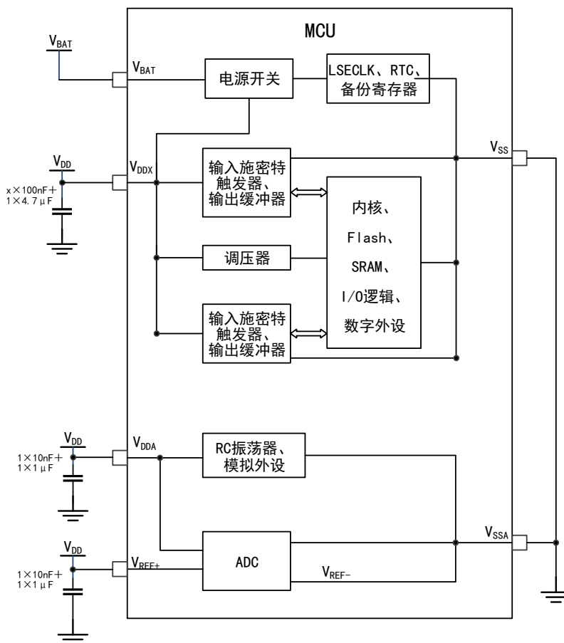
图 7 电源方案
