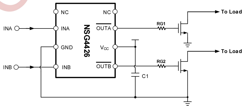
图 10-2 NSG4426 反相典型应用电路图
