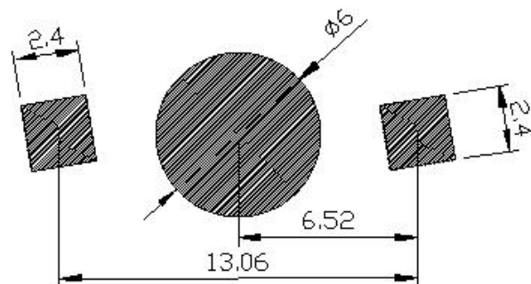
焊盘建议图
