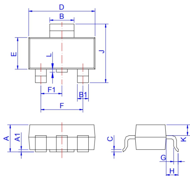
SOT-223-2L
