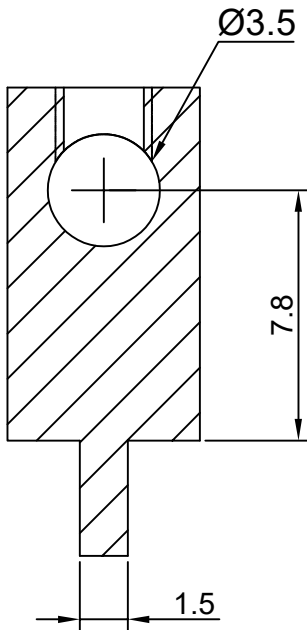
截面 A-A
