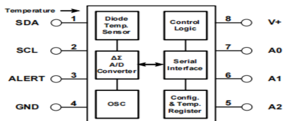
图1 LM75内部各模块示意图
