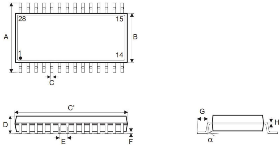
8.7、SOP28（300mil）外形图与封装尺寸
