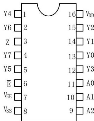
DIP-16/SOP-16/TSSOP-16/QSOP-16
