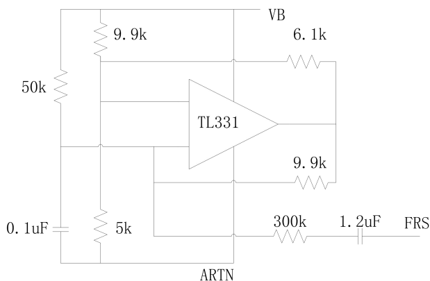
图29 频率抖动
