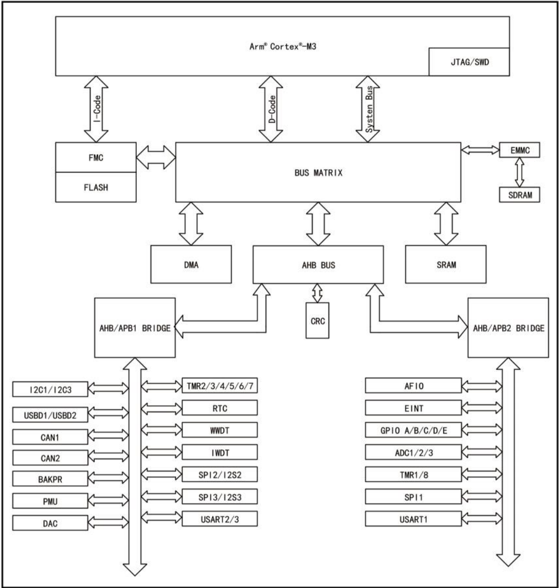
图 6 STM32F103xCTx-TD-合封 SDRAM）系统框图
