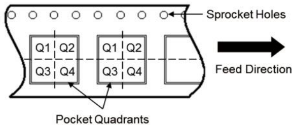
Reel Dimensions
