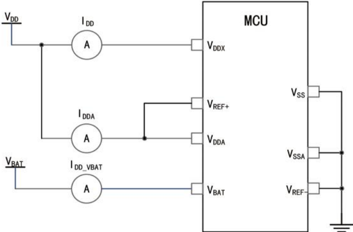
图 11 功耗测量方案
