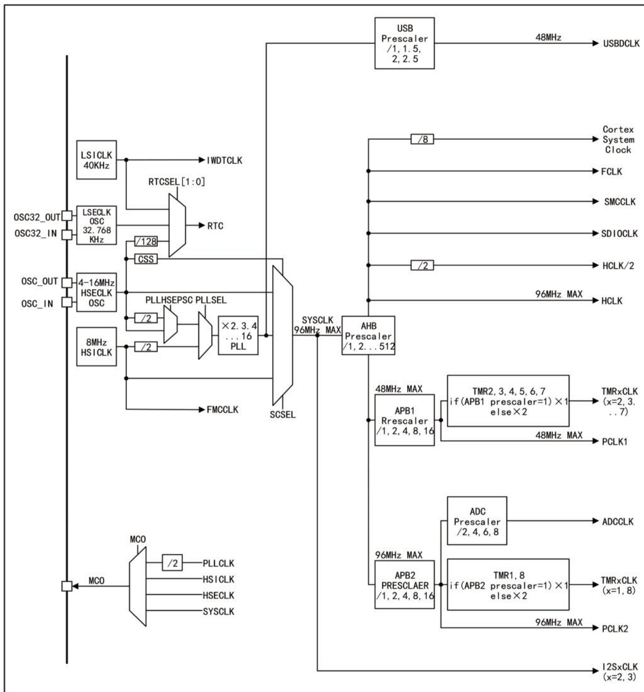
图 7 STM32F103xC 时钟树
