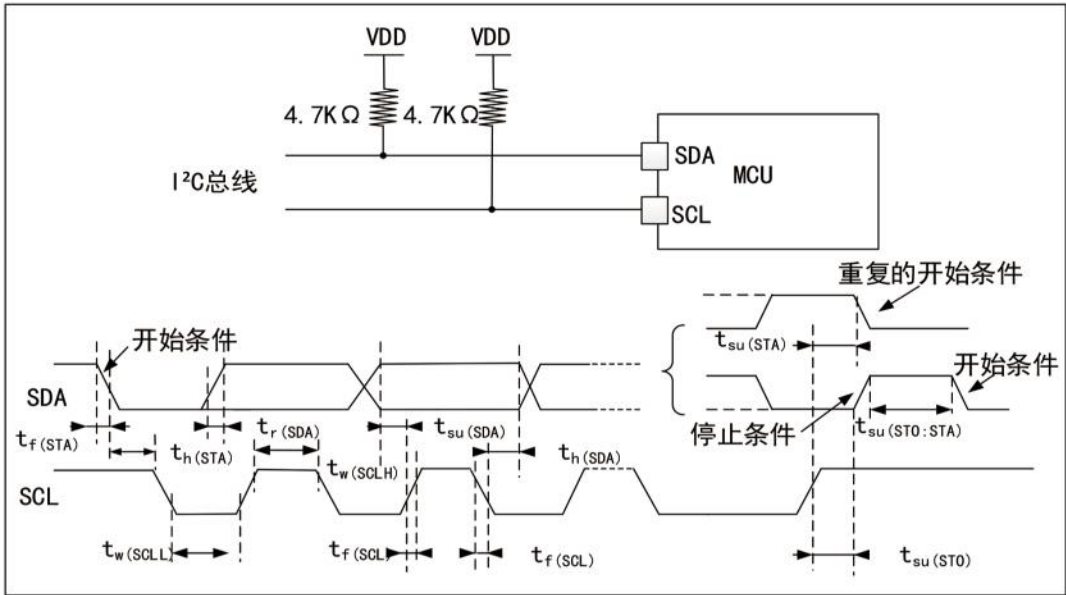
图 13 总线交流波形和测量电路
