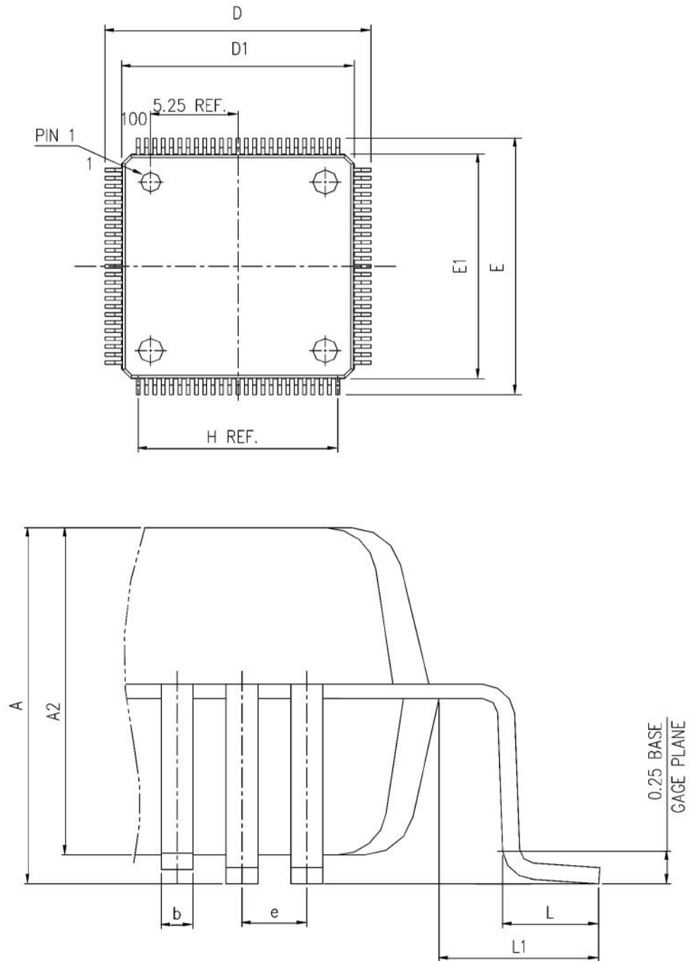
图 17 LQFP100 封装图
