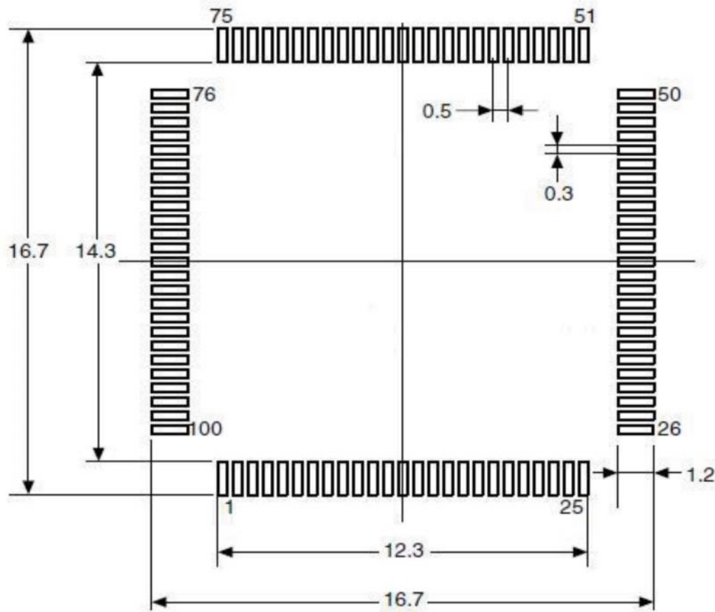
图 18 LQFP100-100 引脚，14×14mm 焊接 Layout 建议
