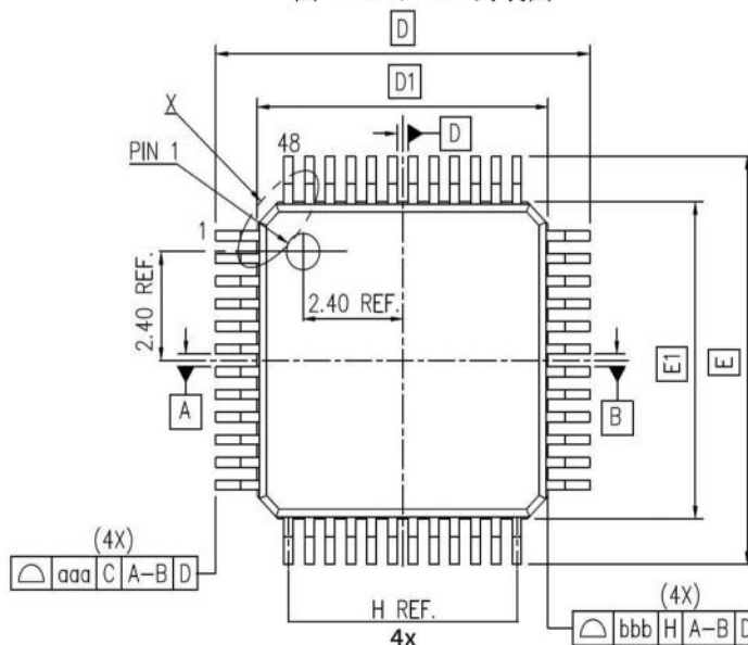
图 23 LQFP48 封装图
