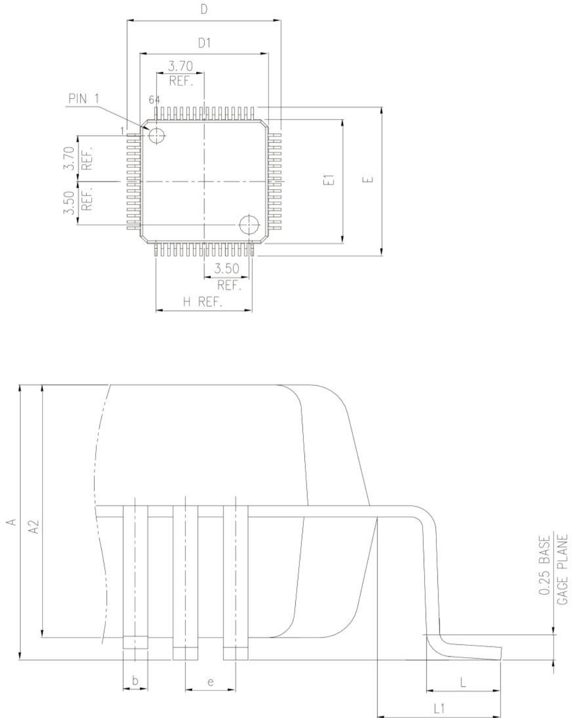
图 20 LQFP64 封装图
