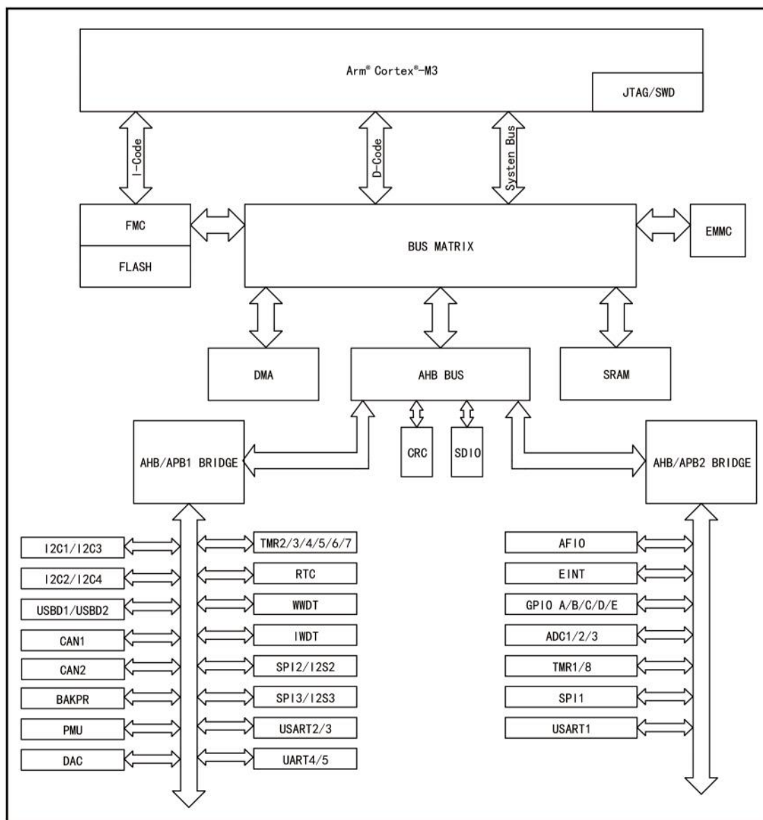
图 5 STM32F103xCTx-TD 系统框图
