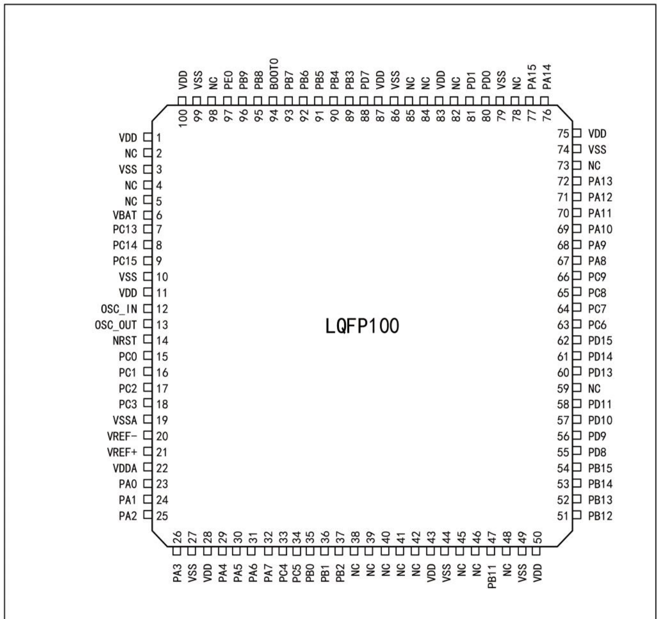
图 1 STM32F103xC-TDtxS（合封 SDRAM）系列 LQFP100 引脚分布图
