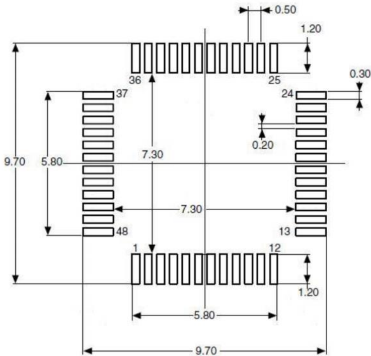
图 24 LQFP48，7×7mm 焊接 Layout 建议
