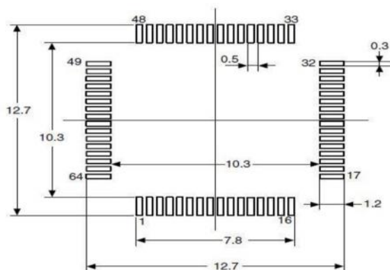
图 21 LQFP64-64 引脚, 10×10mm 焊接 Layout 建议
