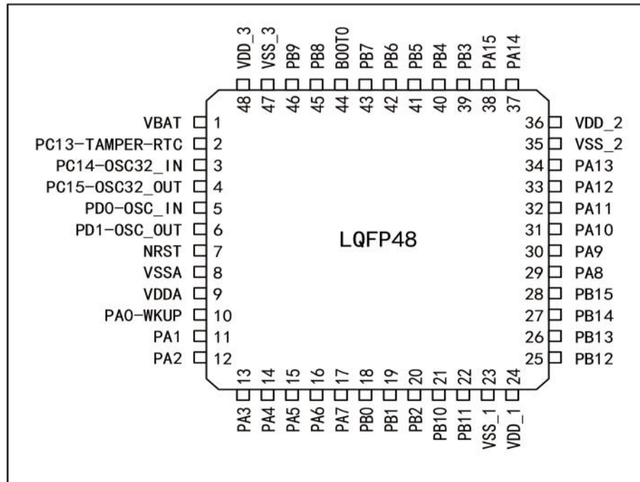
图 4 STM32F103xCTx-TD-TD系列 LQFP48 引脚分布图
