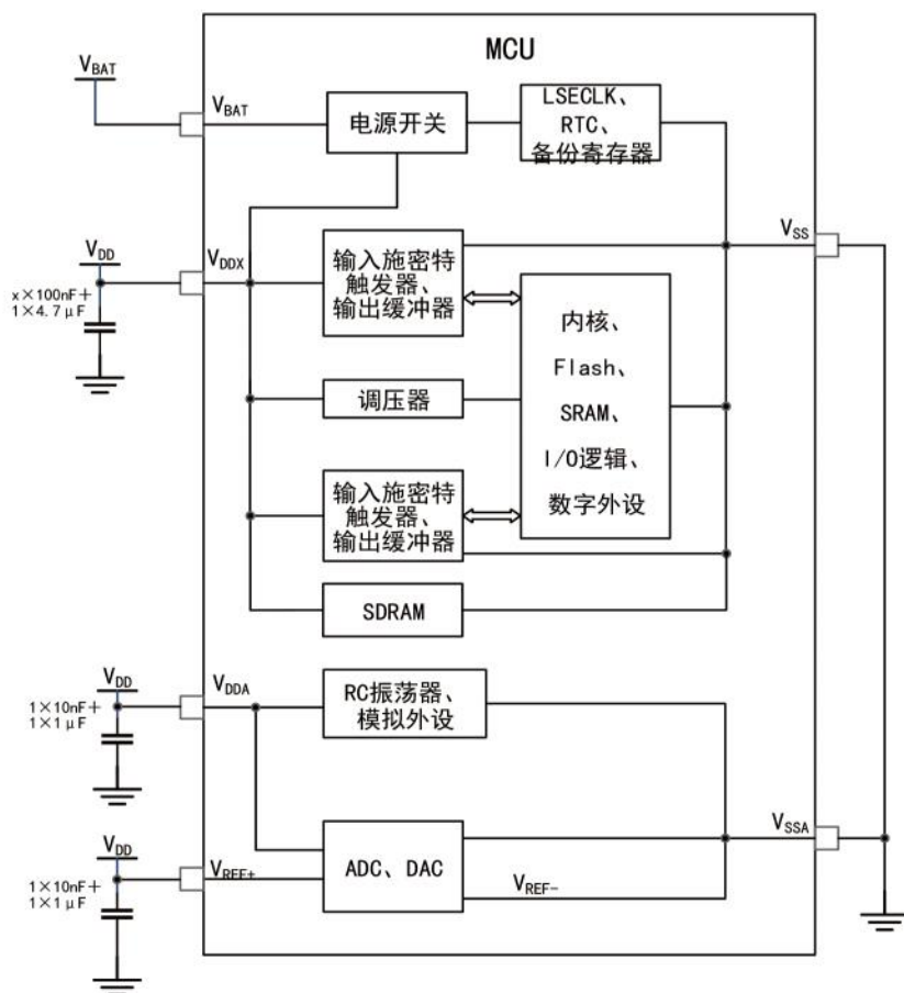
图 8 电源方案
