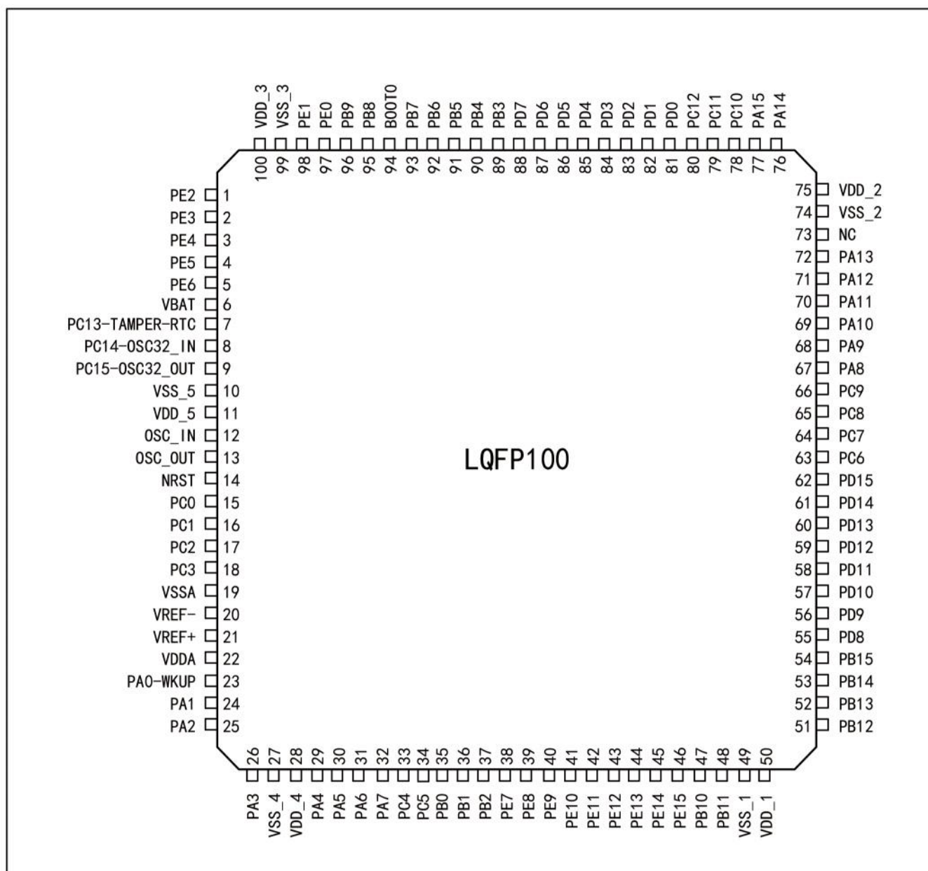
图 2 STM32F103xC-TDTx 系列 LQFP100 引脚分布图
