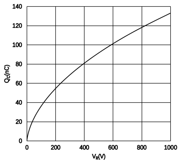
图 4 典型存储电荷与反向电压曲线
