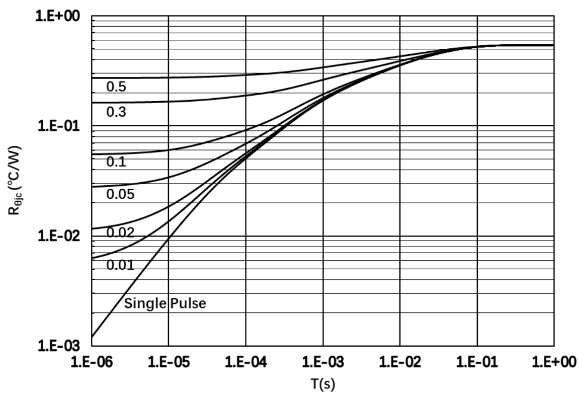
图 7 瞬态热阻抗
