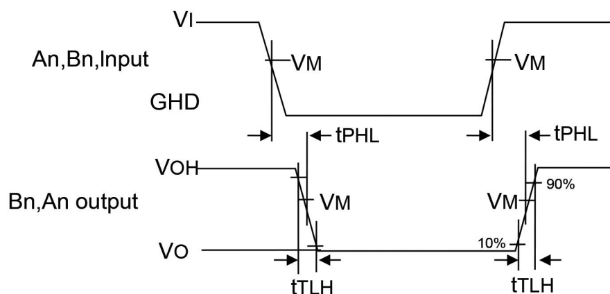
图4、数据输入 (An,Bn) 到数据输出 (Bn,An) 传输延迟及输出转换时间波形
